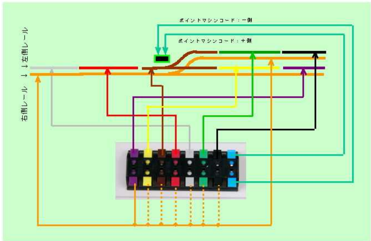
【図1】 端子-レール接続図
